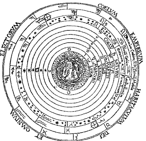
Schemata huius praeaeuae divisionis Sphaerarum.
