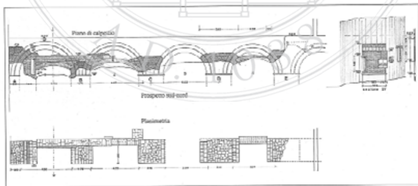
FIG. 3 – Acquedotto e Torre Salustra. In alto: prospetto Sud-Nord; in basso: pianta della porzione di acquedotto (immagine da E. Cirelli 2008).
