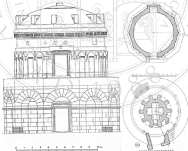
FIG. 19 - Prospetto e piante della cella superiore ed inferiore del Mausoleo (immagini da R. Heidenreich - H. Johannes, 1971; rielaborazione grafica M. Benfatti).
